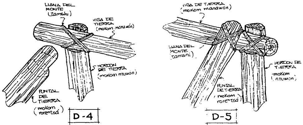
DETALLES DE UNION ENTRE VIGAS INFERIORES Y HORCONES SECUNDARIOS
