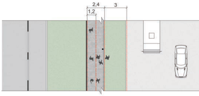
Dimensiones de veredas en la sección de calle.
