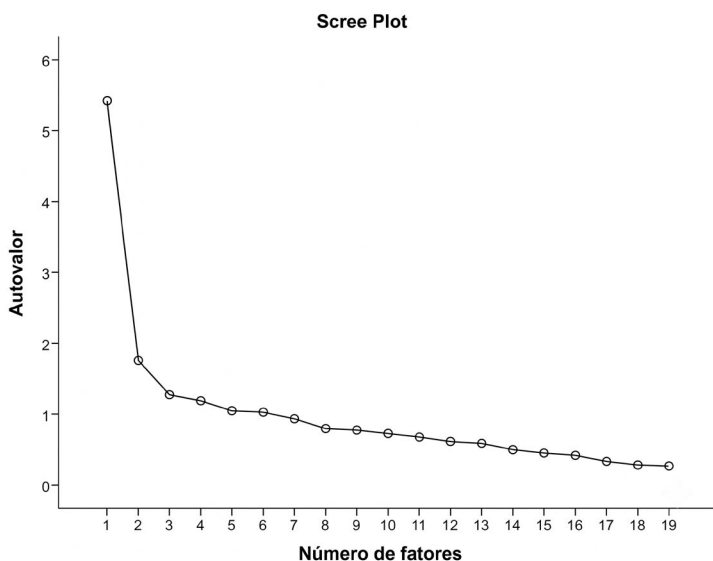
Figura 1. Autovalores empíricos
