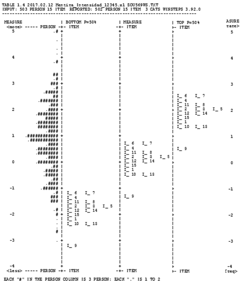
Figura 3. Mapa de Wright para los ítems y sus categorías.
