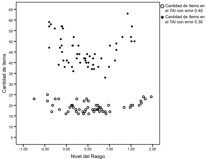
Figura 2. Diagrama de dispersión de la cantidad de ítems necesaria para alcanzar el criterio de parada con respecto a los niveles de rasgo estimados en el TAI de longitud variable con error \leq 0.40 y con error \leq 0.30 .
