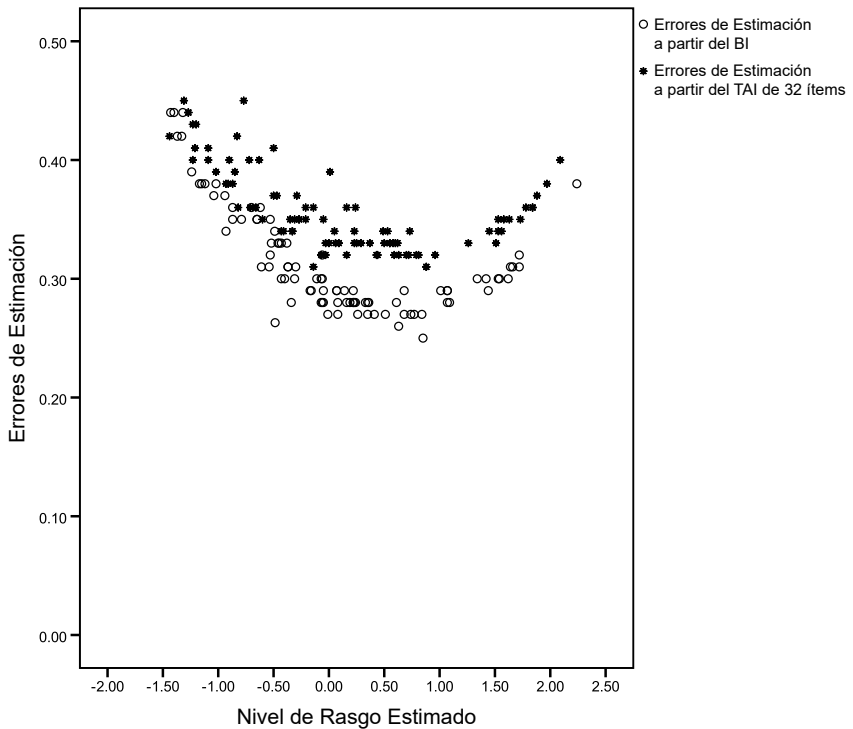
Figura 1. Diagrama de dispersión de los errores de estimación con respecto a los niveles de rasgo estimados a partir de la administración del BI completo y de la administración del TAI de longitud fija de 32 ítems.
