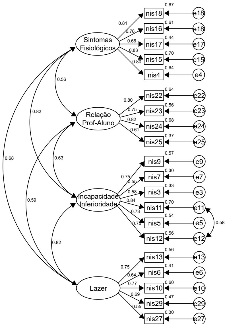
Figura 1. Resultados do modelo fatorial hipotetizado para a Escala de Estresse nos Estudantes (N.I.S.E.S.T.E) (n=244). Porto Alegre, RS. 2013.
